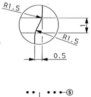
DETTAGLIO A SCALA 5:1
