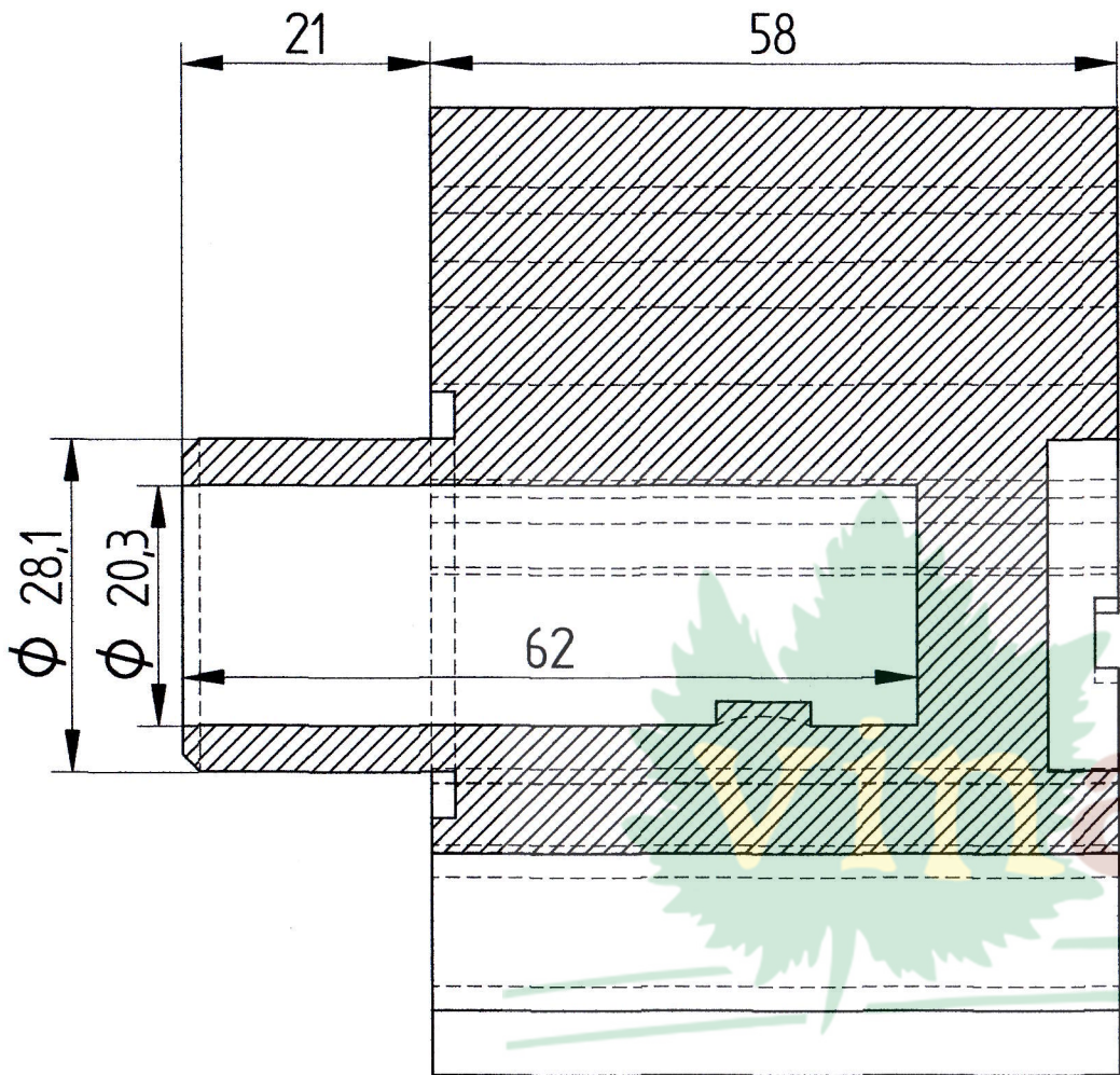
METSZET A-A
